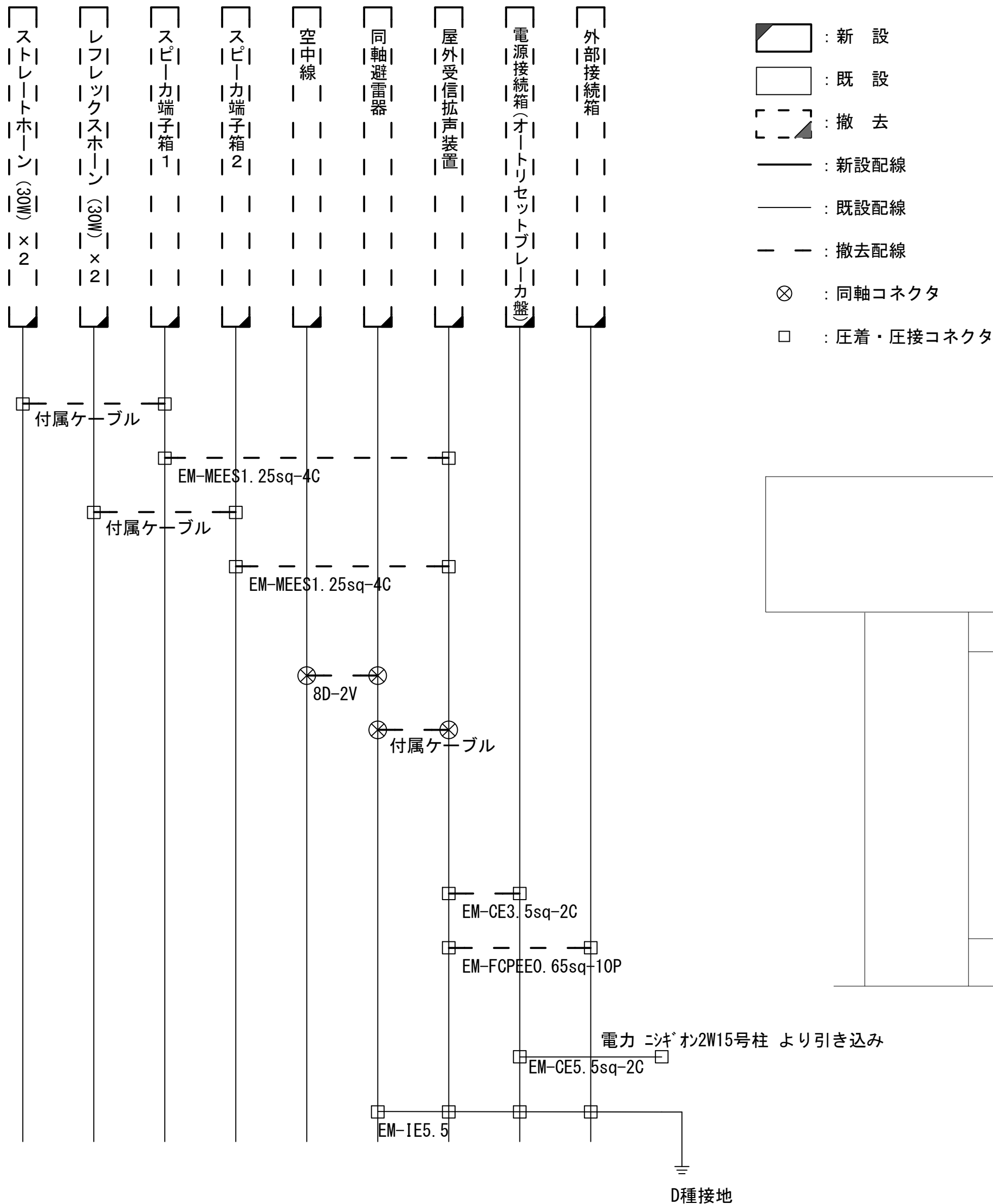
配線系統図
