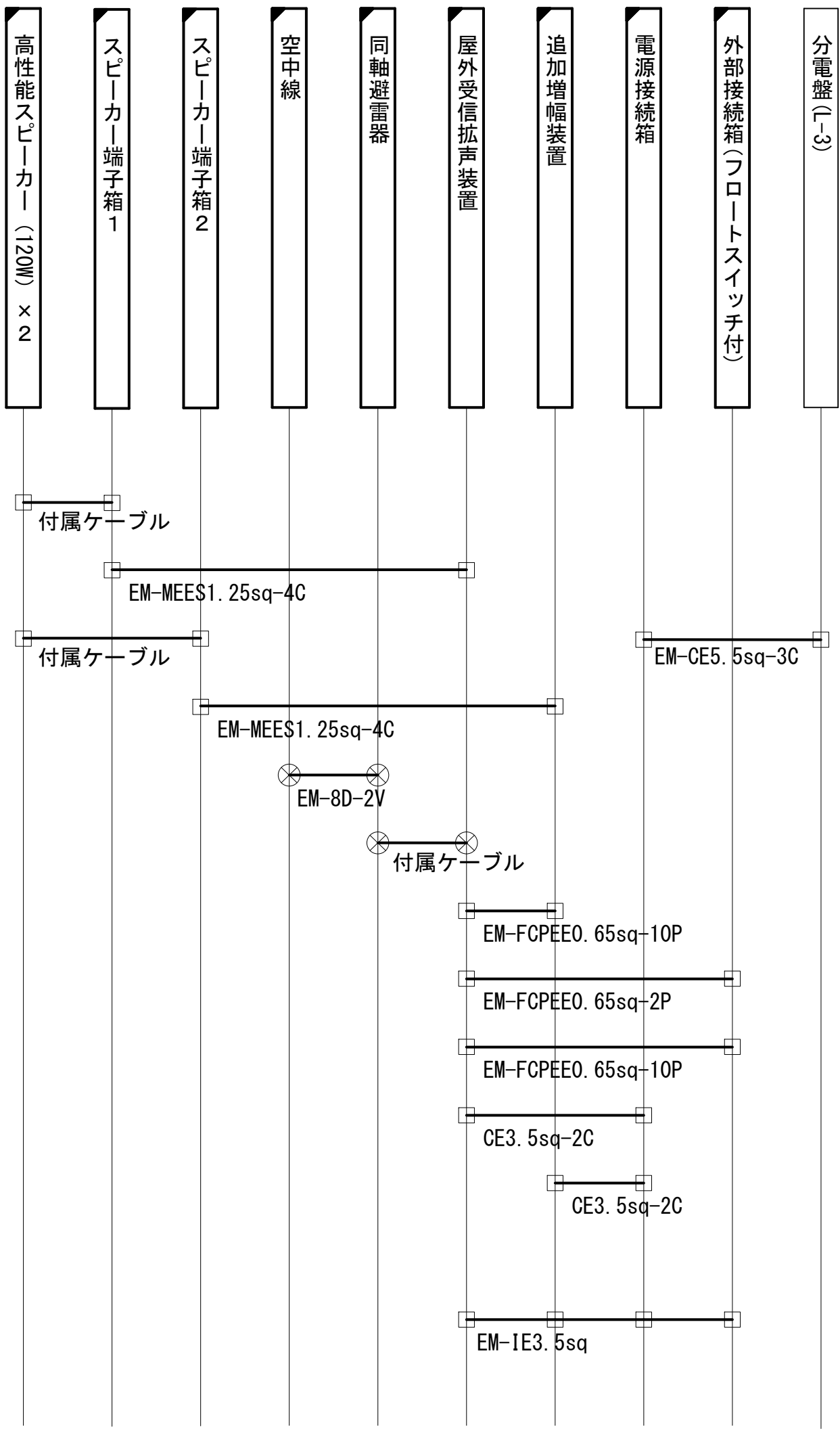
配線系統図
