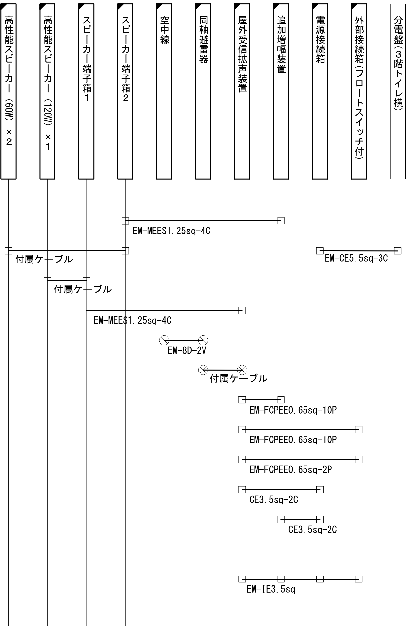
配線系統図
