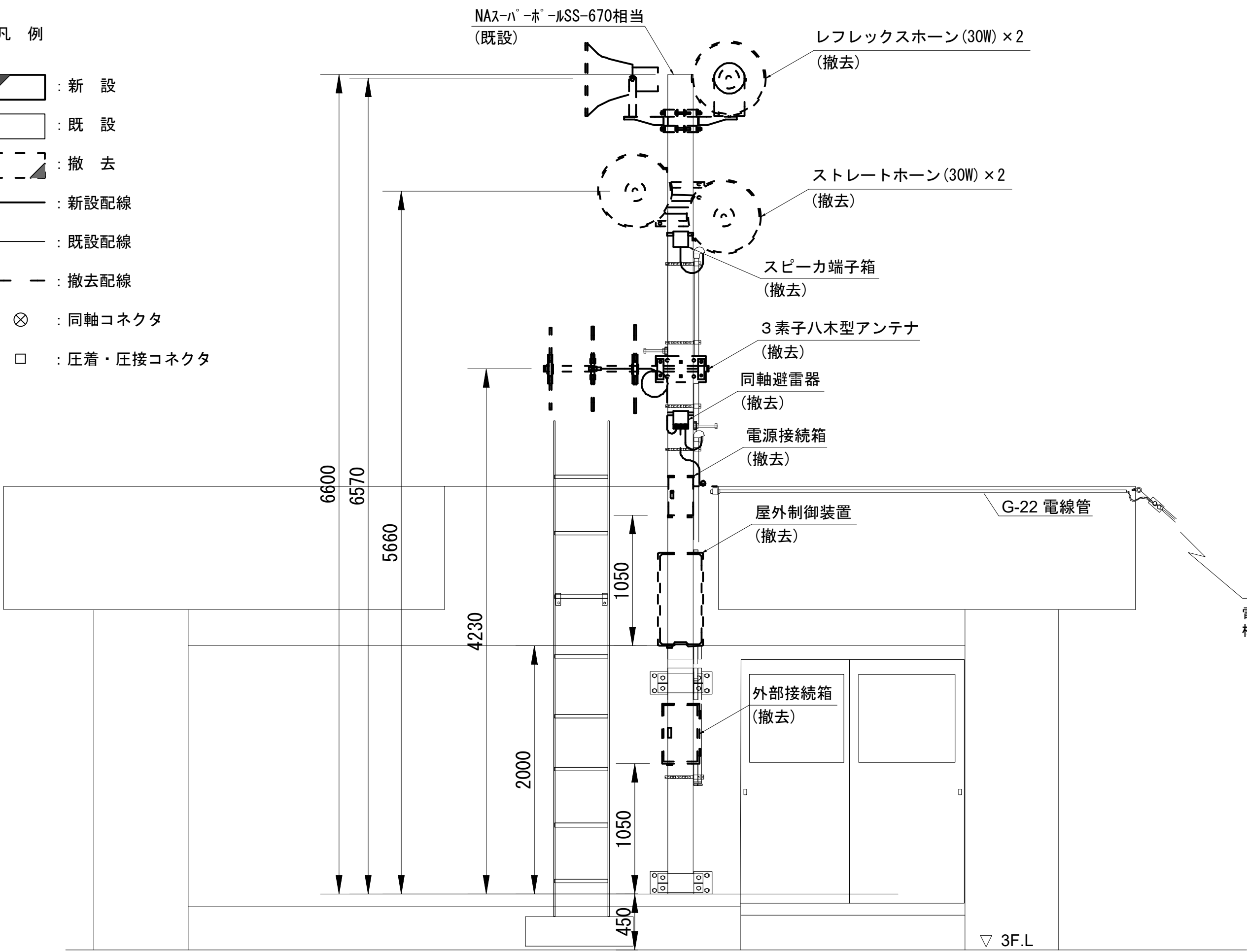
R F 塔屋西向立面
