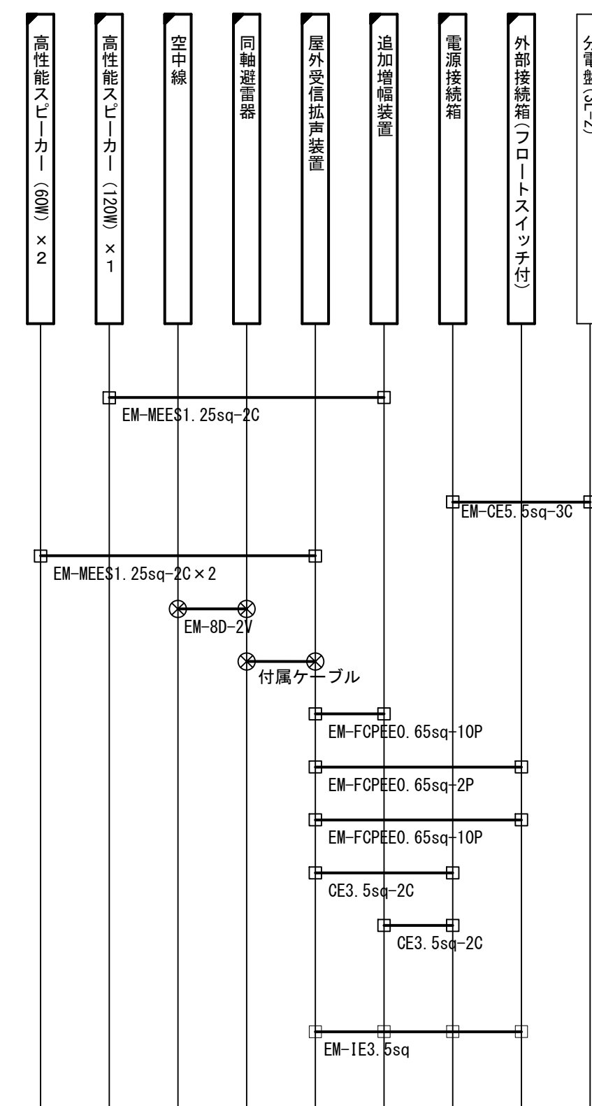
配線系統図
