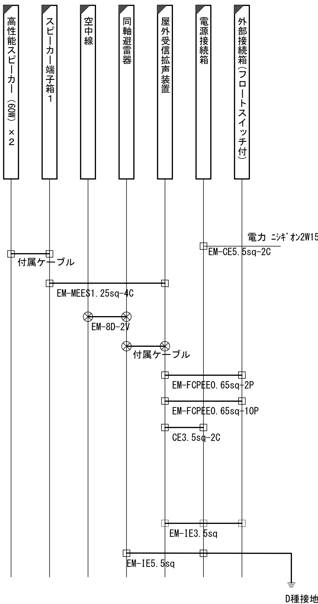
配線系統図
