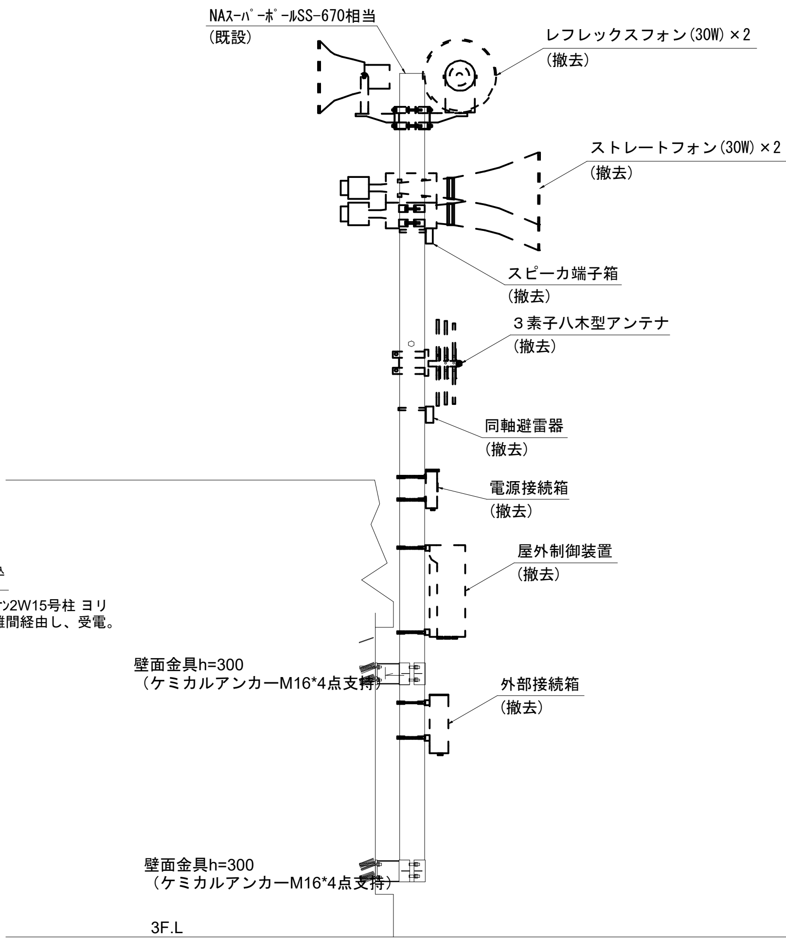
R F 塔屋北向立面
