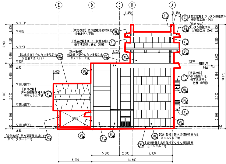
【本館棟】西立面図 S=1/200
