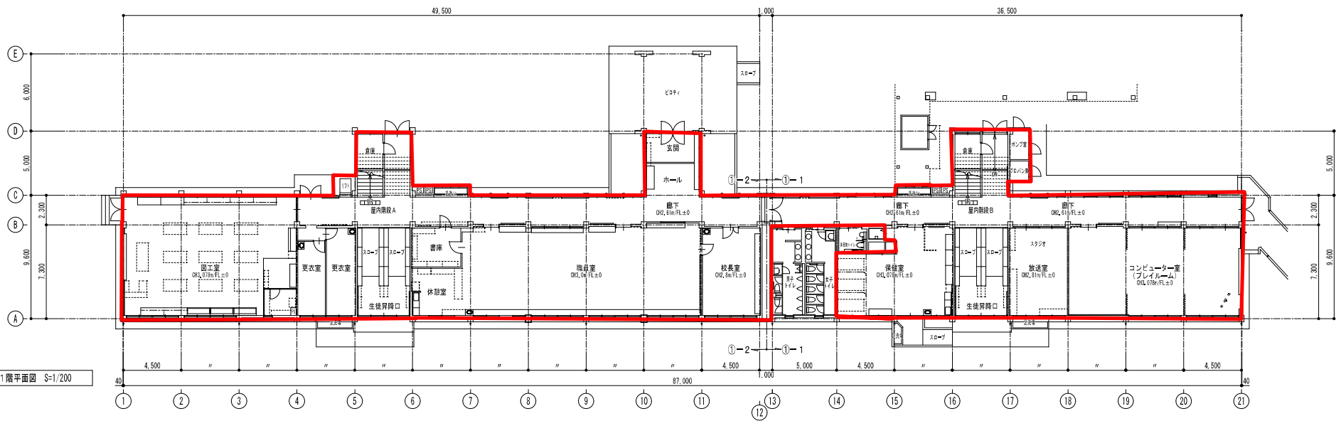
【本館棟】2階平面図 S=1/200
