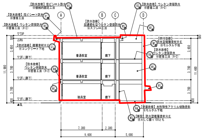
【本館棟】東立面断面図(6通) S=1/200
