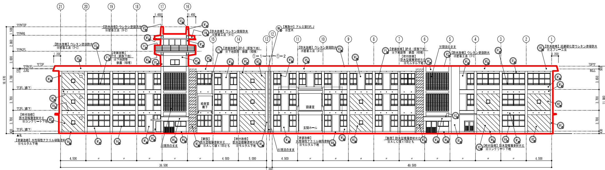
【本館棟】北立面図 S=1/200
