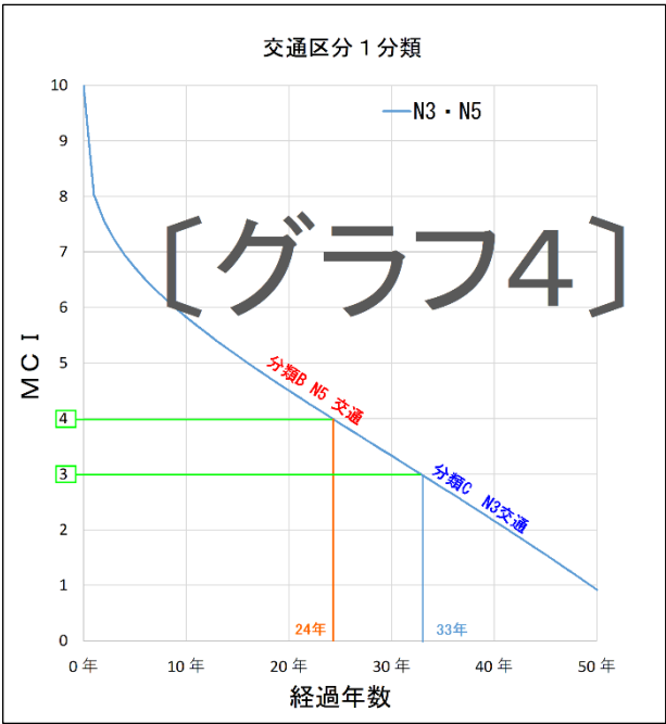
図3.5.2 MCI値より算出した使用目標年数(劣化予測タイプ4)(グラフ4)
