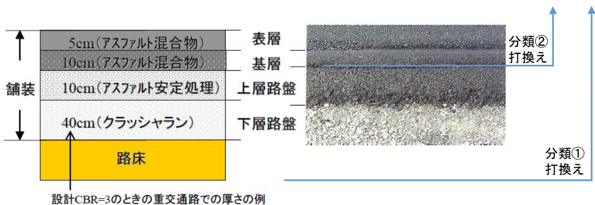
図 4. 2. 1 舗装の修繕対策イメージ図
